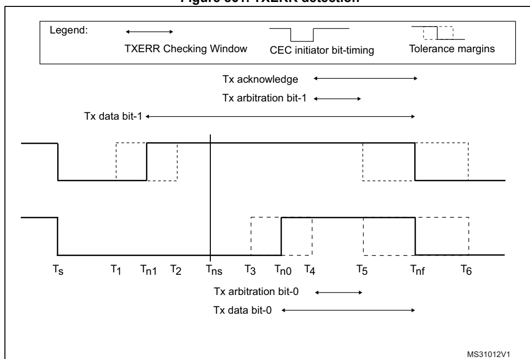
Figure 861. TXERR detection
