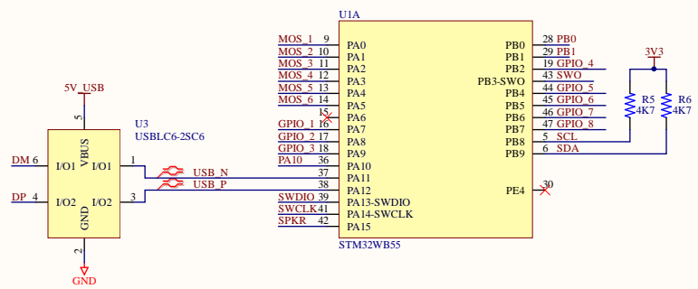
MCU Section
