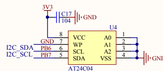
E2数据存储
