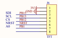
OLED液晶接口
