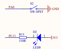
按键和LED灯
